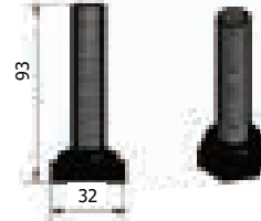
Ürün Kodu : 29093 Ürün Adı : M16x80 Rotil Ayak
