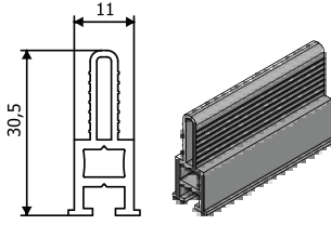
Ürün Kodu : 22046 Ürün Adı : PV4
