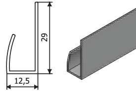
Ürün Kodu : 25022 Ürün Adı : J Profil
