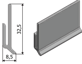
Ürün Kodu : 24054 Ürün Adı : Süpürgelik Plastiği
