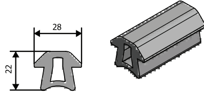
Ürün Kodu : 27006 Ürün Adı : Ray Profili Contası
