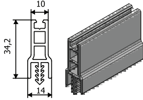
Ürün Kodu : 22015 Ürün Adı : PV-5 Plastik Isı Bariyeri
