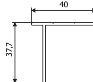
Ürün Kodu : 25009 Ürün Adı : Pencere T Çıtası 40'lık
