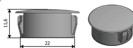
Ürün Kodu : 29191 Ürün Adı : Buzdolabı Yan Kapak Tapası
