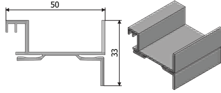
Ürün Kodu : 24005 Ürün Adı : Gövde Profili
