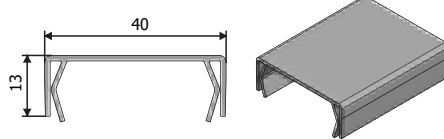
Ürün Kodu : 24018 Ürün Adı : 40mm Poliüretan Gövde Plastiği
