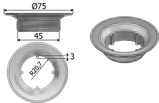
Ürün Kodu : 29195 Ürün Adı : 40'luk Su Gideri Üst Enjeksiyon
