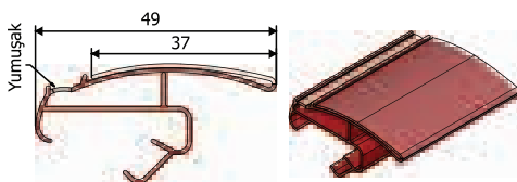
Ürün Kodu : 24087 Ürün Adı : 40mm Bombeli Sallanır Raf Etiketlik
