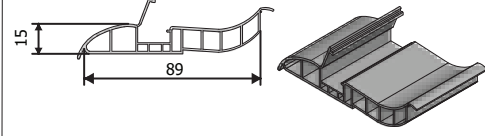
Ürün Kodu : 25048 Ürün Adı : Zemin Hijyen Profili
