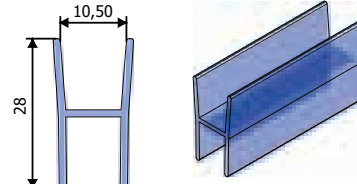
Ürün Kodu : 21006 Ürün Adı : 10x12 Cam Profili
