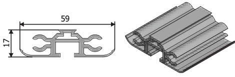
Ürün Kodu : 24057 Ürün Adı : Aydınlatma Birleştirme Profil
