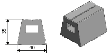
Ürün Kodu : 27005 Ürün Adı : Forklift Bariyeri
