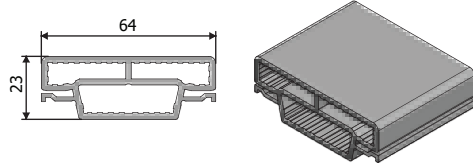
Ürün Kodu : 24036 Ürün Adı : Sütük Gövde Birleştirme
