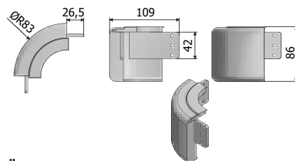
Ürün Kodu : 29208 Ürün Adı : Tampon Köşe Enjeksiyon
