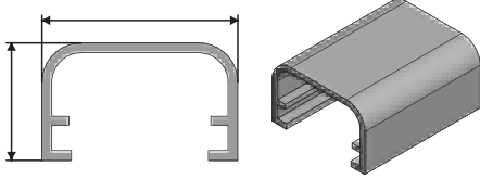
Ürün Kodu : 24051 Ürün Adı : Isıcam Profili Çift Tırnaklı
