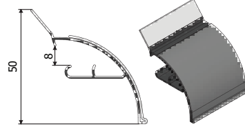
Ürün Kodu : 24093 Ürün Adı : 50mm Bombeli Etiketlik Profil
