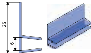
Ürün Kodu : 21009 Ürün Adı : F Profil
