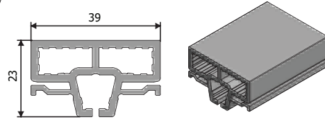
Ürün Kodu : 24029 Ürün Adı : Sütük Gövde Birleştirme Erkek
