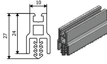
Ürün Kodu : 22014 Ürün Adı : PV-4 Plastik Isı Bariyeri
