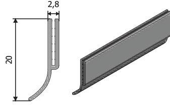
Ürün Kodu : 24038-2 Ürün Adı : Radüslü Süpürgelik Profili Coex
