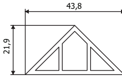
Ürün Kodu : 25003 Ürün Adı : Eşik Üçgen Profil 40x40
