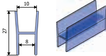
Ürün Kodu : 21005 Ürün Adı : 8x10 Cam Profili
