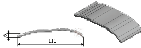
Ürün Kodu : 27002 Ürün Adı : PVC Branda Profili
