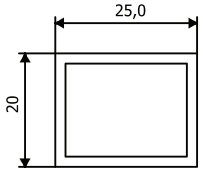
Ürün Kodu : 22027 Ürün Adı : 20x25 Kutu Profil
