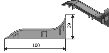
Ürün Kodu : 29148 Ürün Adı : Zemin Hijyen Sağ Bitim
