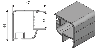
Ürün Kodu : 24086 Ürün Adı : Kola Dolabı Kapı Profili 21mm
