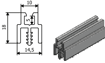
Ürün Kodu : 22013 Ürün Adı : PV-3 Plastik Isı Bariyeri
