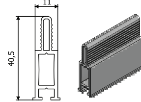
Ürün Kodu : 22047 Ürün Adı : PV5
