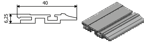
Ürün Kodu : 22032 Ürün Adı : Plastik Profil Alüminyuma Geçme
