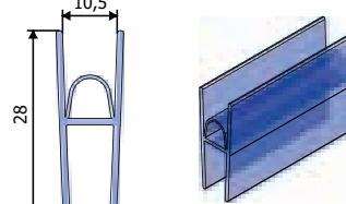
Ürün Kodu : 21010 Ürün Adı : 8x10 Balonlu Cam Çıtası
