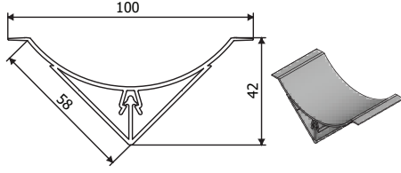
Ürün Kodu : 25031 Ürün Adı : 100'lük Soğuk Oda Hijyen Profili
