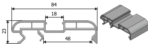
Ürün Kodu : 24111 Ürün Adı : Tampon Profili
