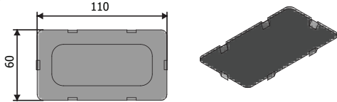
Ürün Kodu : 29122 Ürün Adı : Sütlük Arka Üfleme Kapama Plastiği
