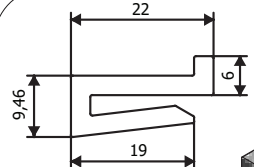
Ürün Kodu : 25017 Ürün Adı : Yan Profil
