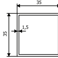
Ürün Kodu : 22089 Ürün Adı : 35x35 Kutu Profil
