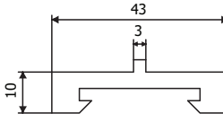
Ürün Kodu : 25016 Ürün Adı : Orta Profil
