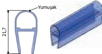
Ürün Kodu : 21007 Ürün Adı : Balon Fitol 8mm
