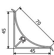
Ürün Kodu : 25014 Ürün Adı : 70'lık Soğuk Oda Hijyen Profili
