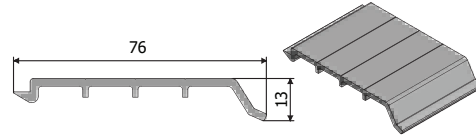
Ürün Kodu : 24076-2 Ürün Adı : Yazar Kasa Tampon Profili Çizgili Düz
