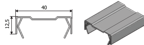
Ürün Kodu : 24066 Ürün Adı : 40mm Poliüretan Gövde Kapama
