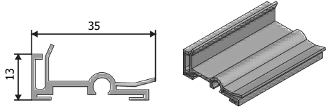
Ürün Kodu : 24016 Ürün Adı : Kapi Cam Profili
