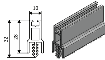
Ürün Kodu : 22016 Ürün Adı : PV-3 Isı Bariyeri Plastik
