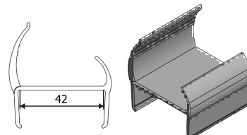
Ürün Kodu : 27008 Ürün Adı : PVC Kapı İzolasyon Plastiği 42mm
