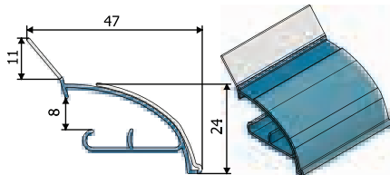
Ürün Kodu : 24069 Ürün Adı : 40mm Etiketlik Profil Bombeli
