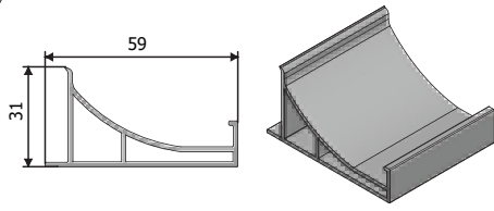
Ürün Kodu : 24025 Ürün Adı : Sütük Dolabı Üfleme Plastiği
