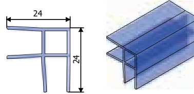
Ürün Kodu : 21004 Ürün Adı : 90 Derece Köşe Profili
