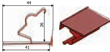
Ürün Kodu : 24007 Ürün Adı : 40mm Etiketlik Profil
