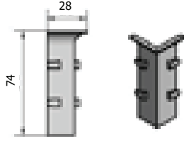
Ürün Kodu : 25006 Ürün Adı : Süpürgelik İç Köşe
