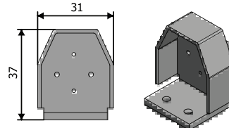
Ürün Kodu : 29040 Ürün Adı : Florasan Koruma Kapağı Üst
