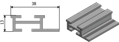
Ürün Kodu : 24029-3 Ürün Adı : Soğuk Oda Kapı Çıtası
