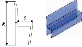
Ürün Kodu : 21001 Ürün Adı : 8mm Cam Çıtası
